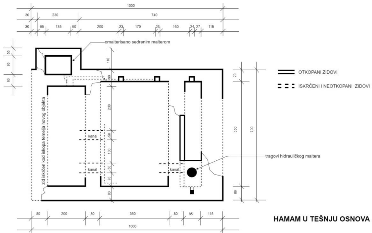
Sl. 17. Dimenzije hamama u Tešnju (izradili inž. Admir Agić i Ana Jozić Agić) 146
