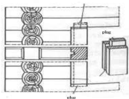
Ilustracija 21. Detalji ukrucenja zidova
