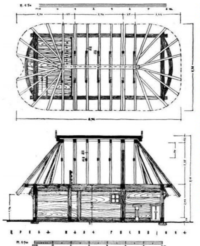
Ilustracija 19. Nacrt crkve u Malom Blašku
