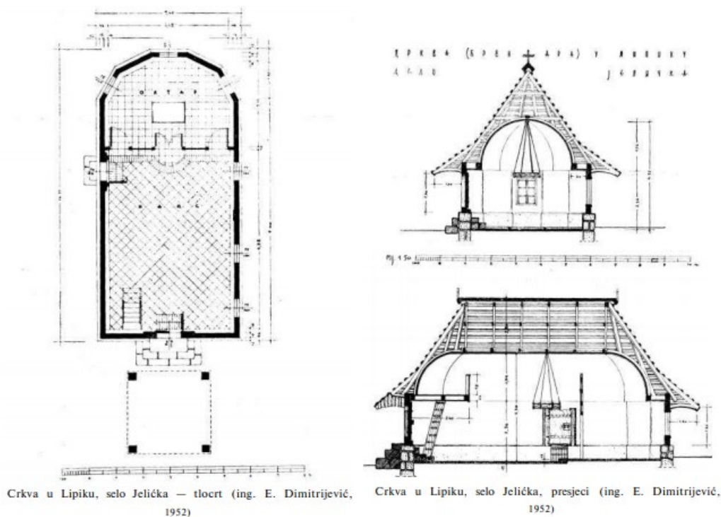
Ilustracija 33. Tlocrt i presjek crkve u Jeličkoj
