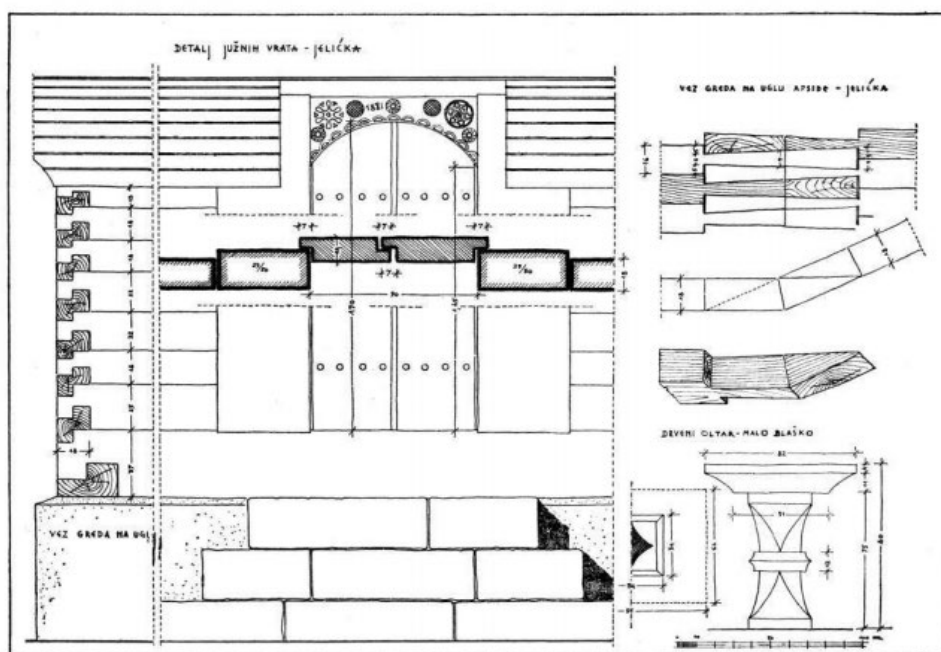
Detalji sa crkve u Jelički i Malom Blaškom (ing. E. Dimitrijević, 1952)
