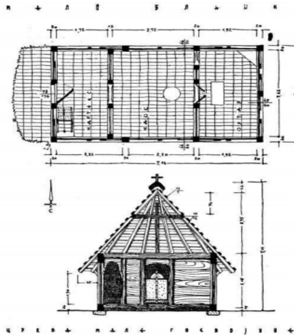
Ilustracija 18. Nacrt crkve u Malom Blašku
